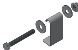
ENTRETOISE HDS 4530
